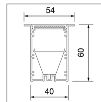
40 x 60 mm, mit Kragen
